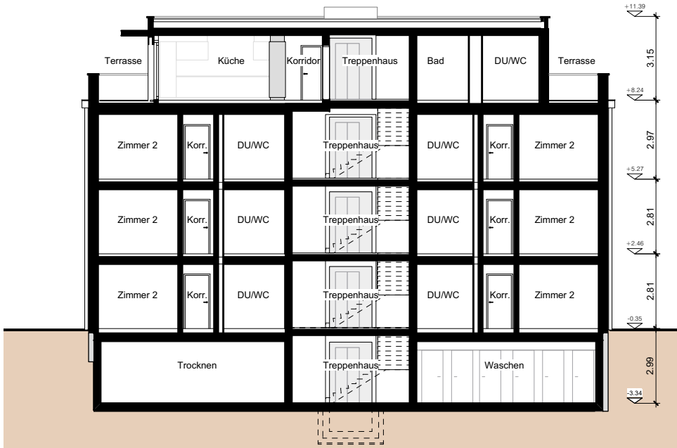
SCHNITT 1-1
